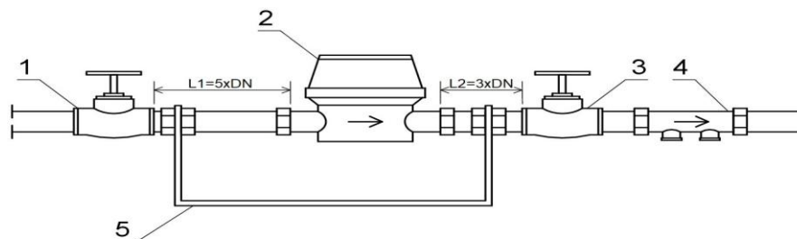
Schemat zestawu wodomierzowego - rysunek nr 1
